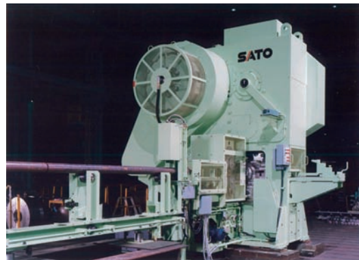
8000kN精密鍛造素材切断機
