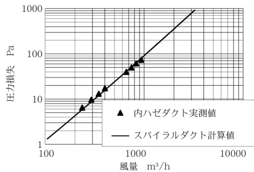
図5 内ハゼダクトの圧力損失(計算値との比較)
